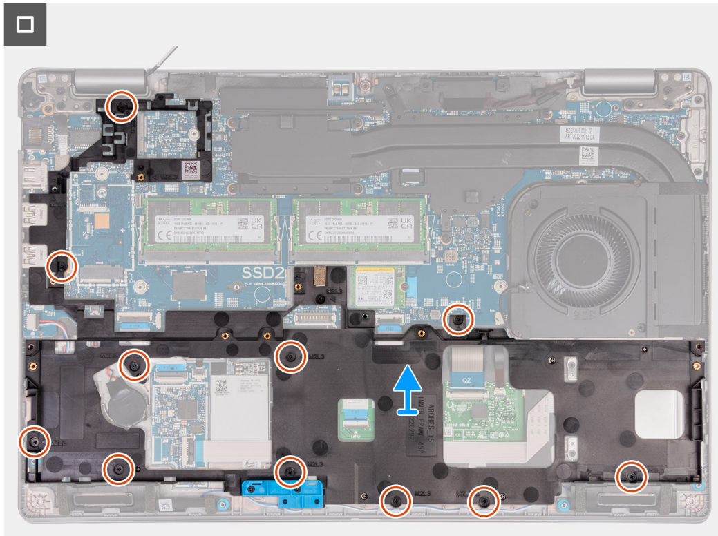
Abbildung 3. Entfernen des inneren Rahmens
