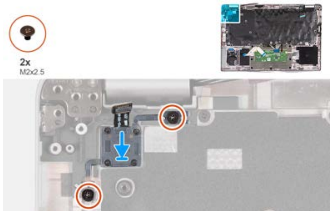
Abbildung 60. Einbauen der Netzschalterplatine
