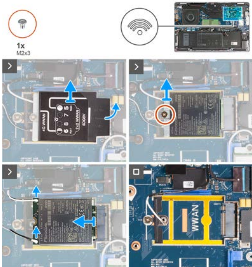
Abbildung 12. Entfernen der WWAN-Karte (bei Computern mit 4G-Karte)
