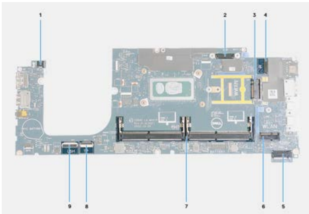
Abbildung 53. Systemplattenanschlüsse
