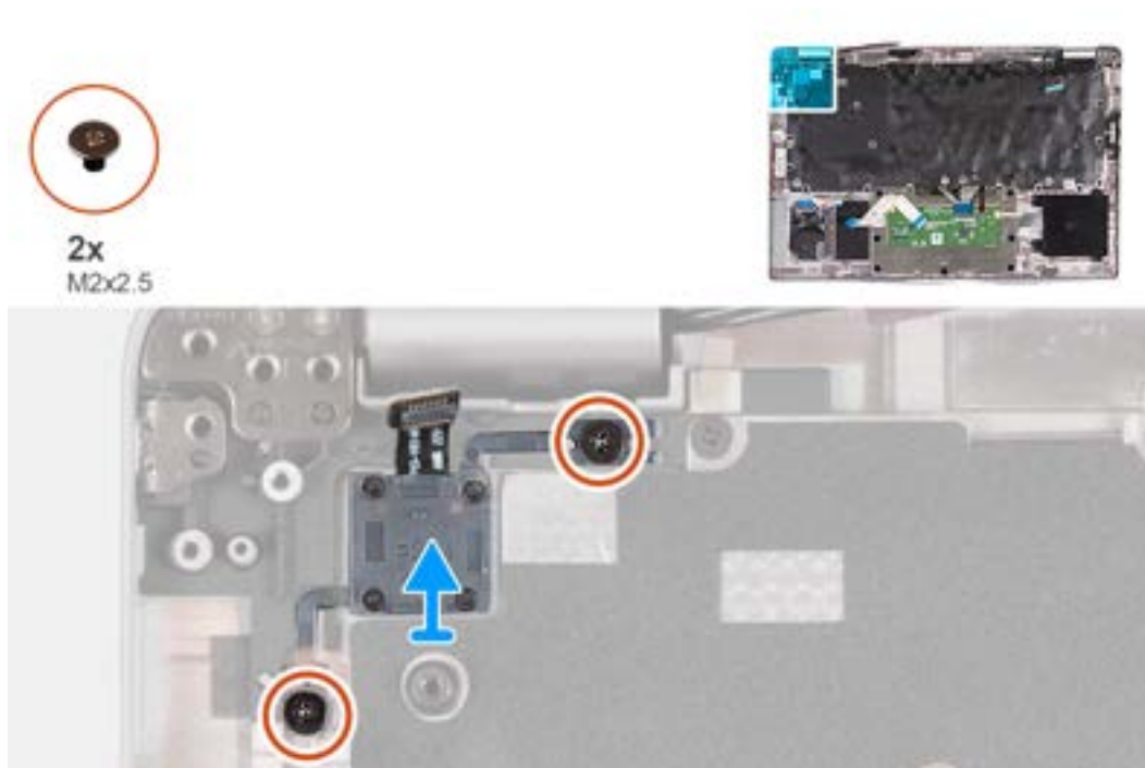
Abbildung 59. Entfernen der Netzschalterplatine
