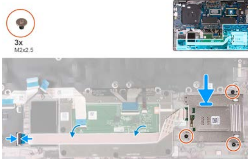
Abbildung 58. Einbauen des Smartcardlesegeräts
