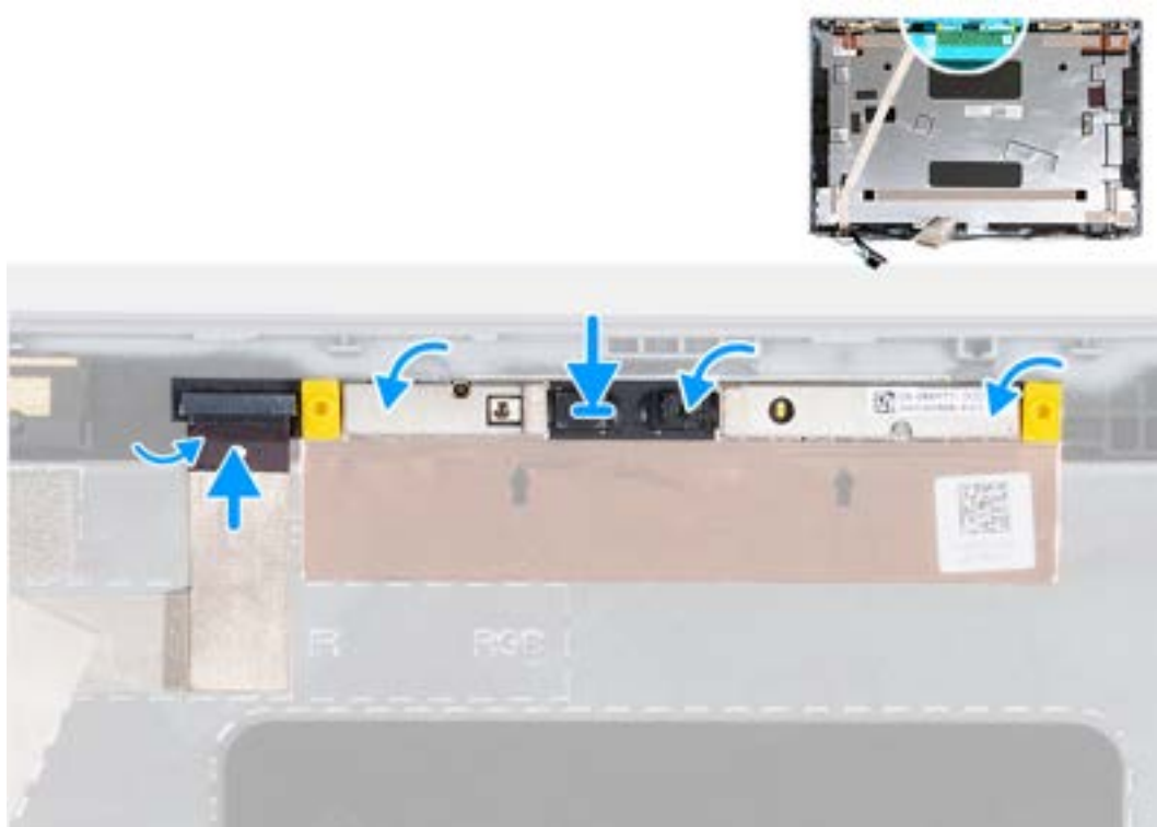
Abbildung 46. Einbauen des Kameramoduls
