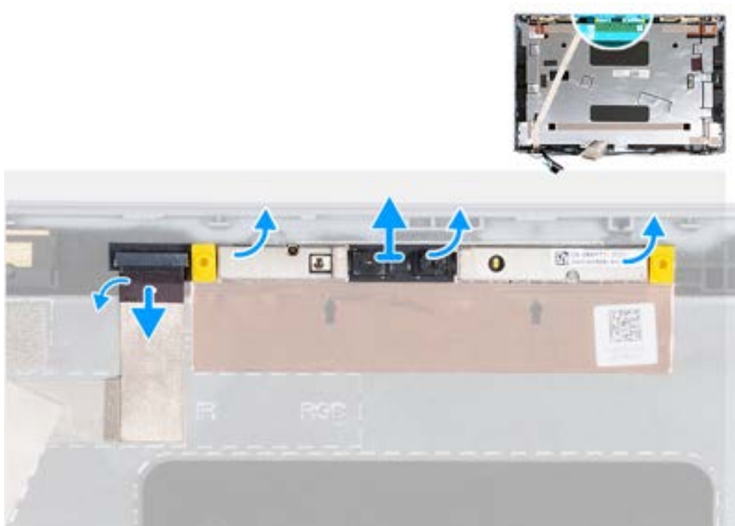
Abbildung 45. Entfernen des Kameramoduls
