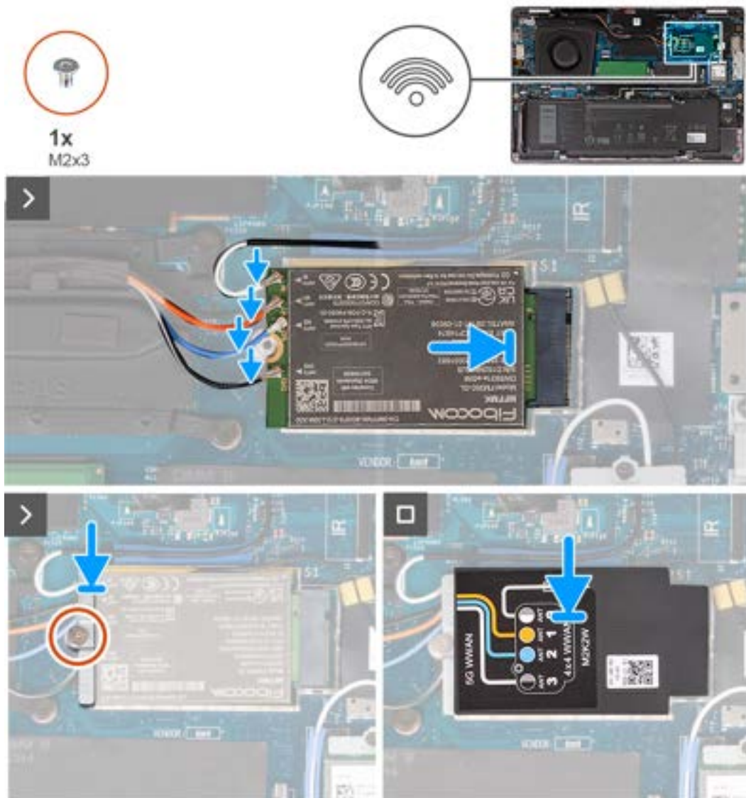
Abbildung 15. Einbauen der WWAN-Karte (bei Computern mit 5G-Karte)
