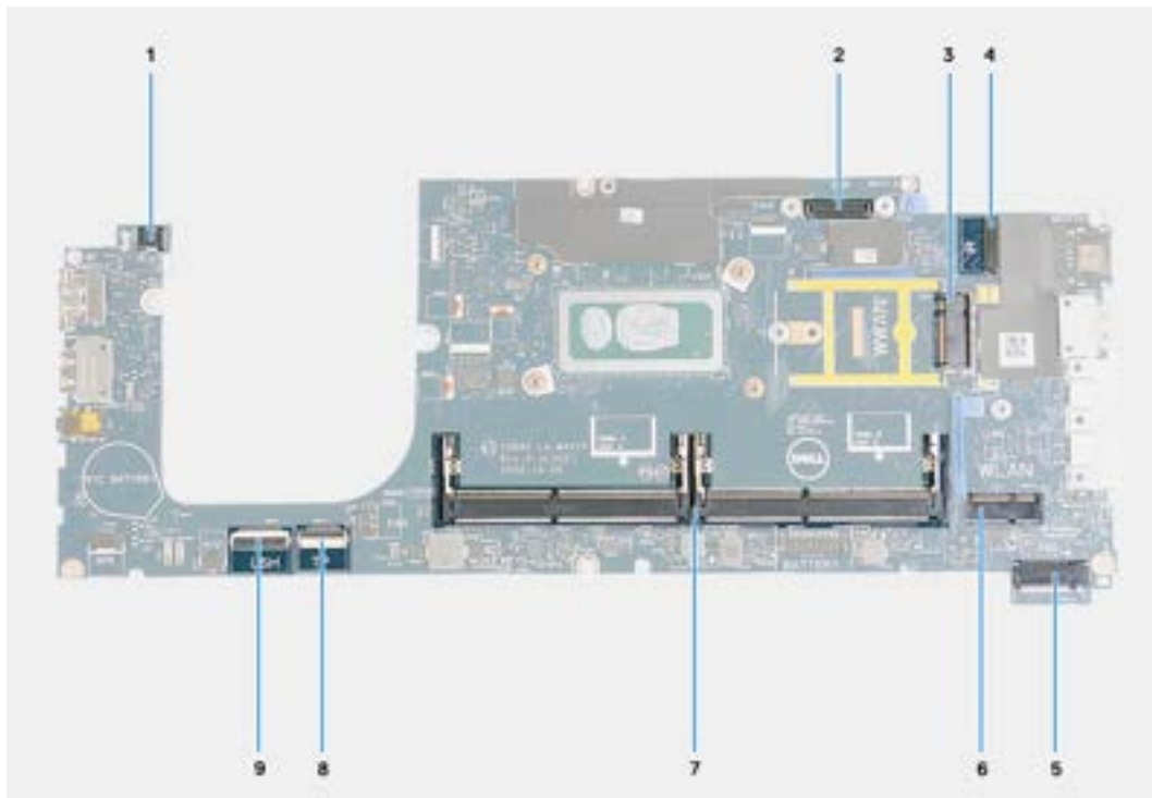
Abbildung 55. Systemplattenanschlüsse
