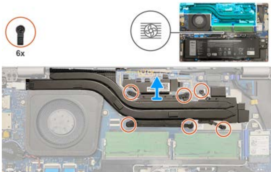
Abbildung 27. Kühlkörper entfernen
