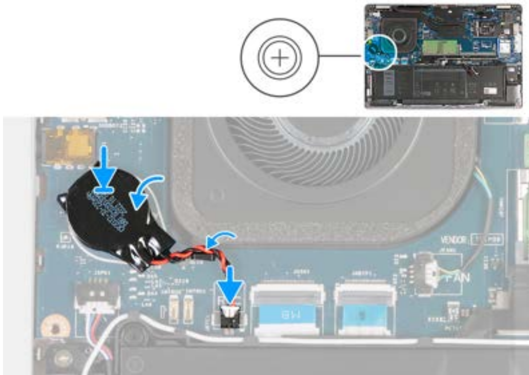
Abbildung 21. Einsetzen der Knopfzellenbatterie
