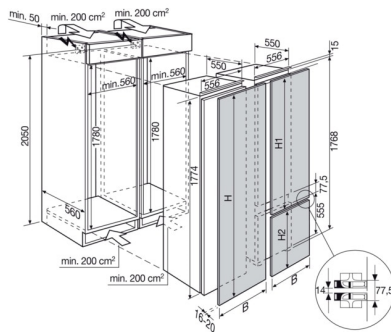
IK3318C und IK2708BZ – Euro-Einbau Möbelfronten auf Gerätetüren verschraubt
