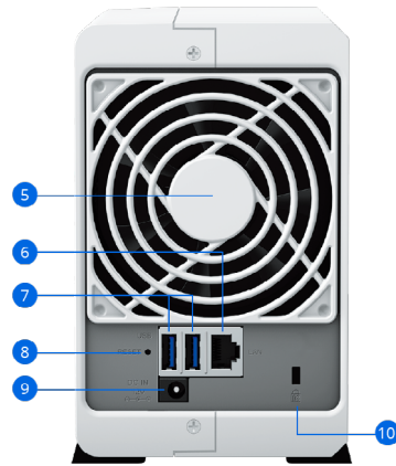
DS223j (Rückseite)
