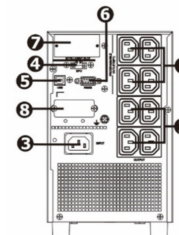
Abbildung 15: Rückansicht ZINTO 1500
