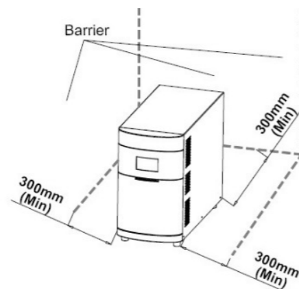
Abbildung 3: ZINTO 800 – 3000 erforderliche Abstände
