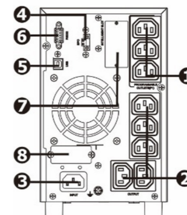
Abbildung 14: Rückseite ZINTO 800/1000
