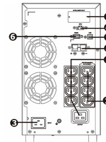
Abbildung 17: Rückansicht ZINTO 3000
