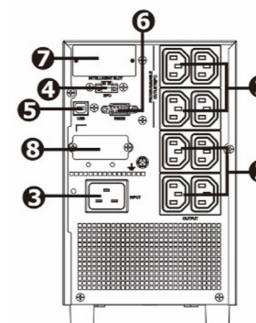
Abbildung 16: Rückansicht ZINTO 2000
