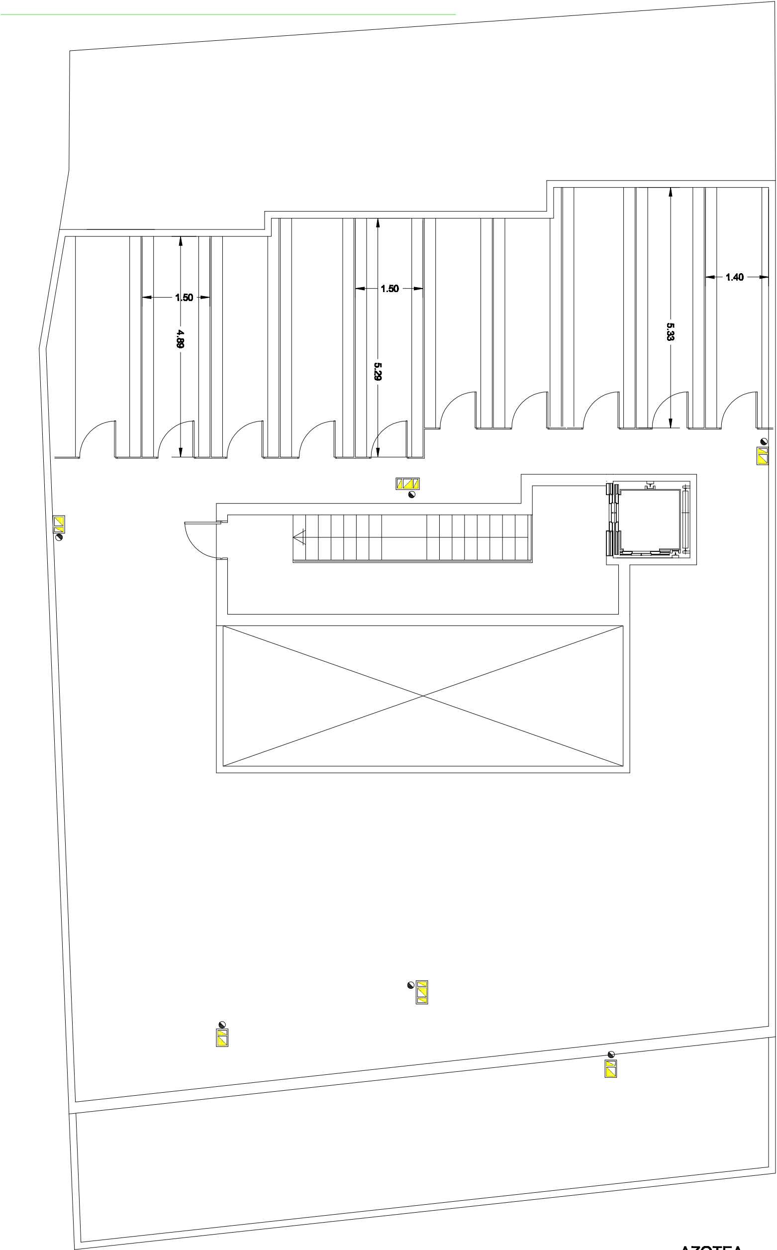
AZOTEA ESCALA 1/100
