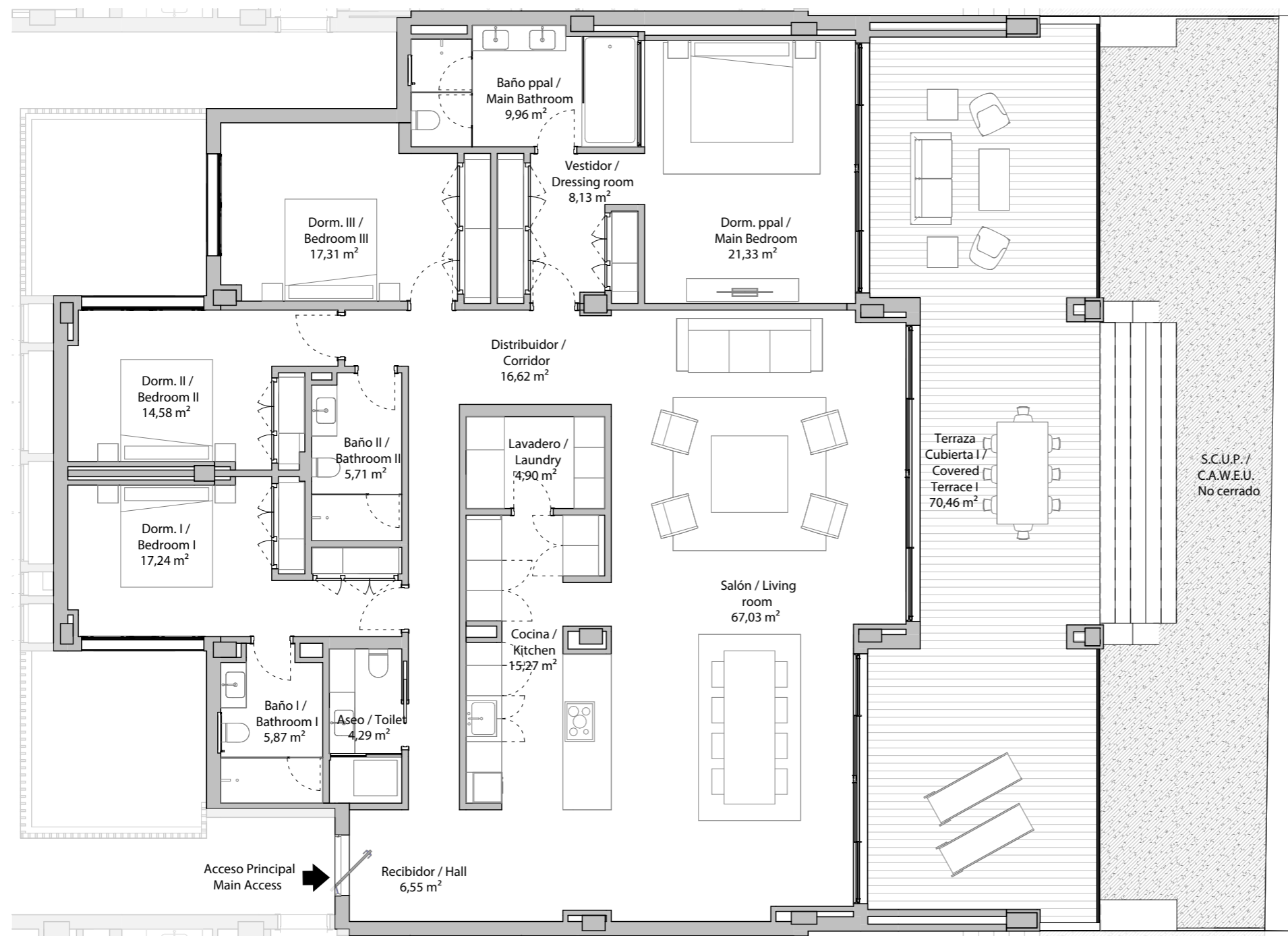
PLANTA VIVIENDA
