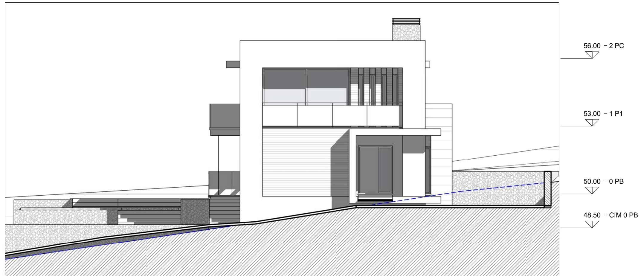
2 Oeste 3 1:100
