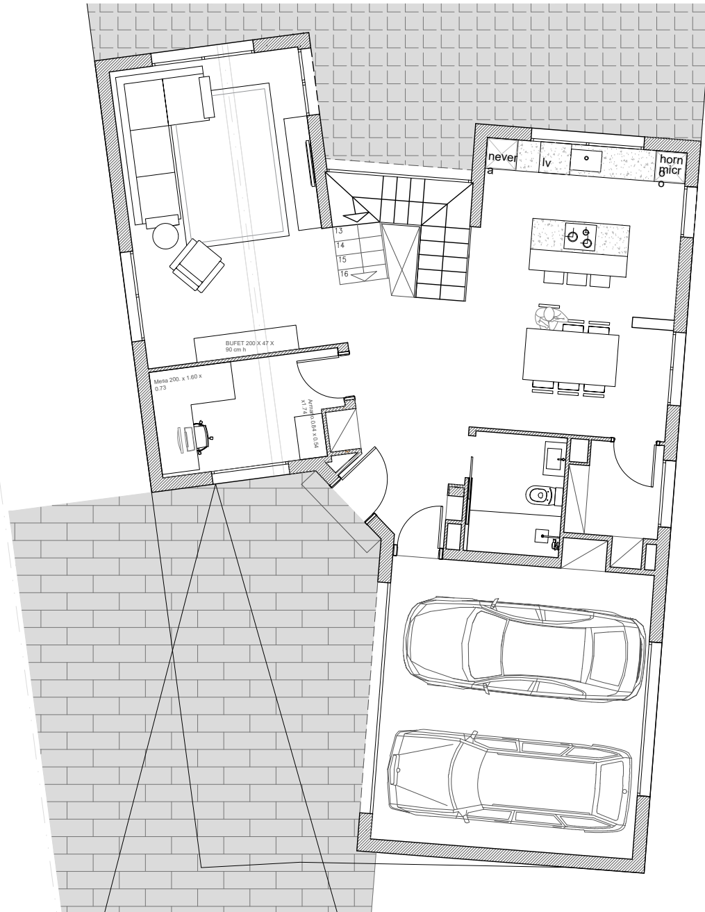
DISTRIBUCIÓN - PLANTA BAJA
