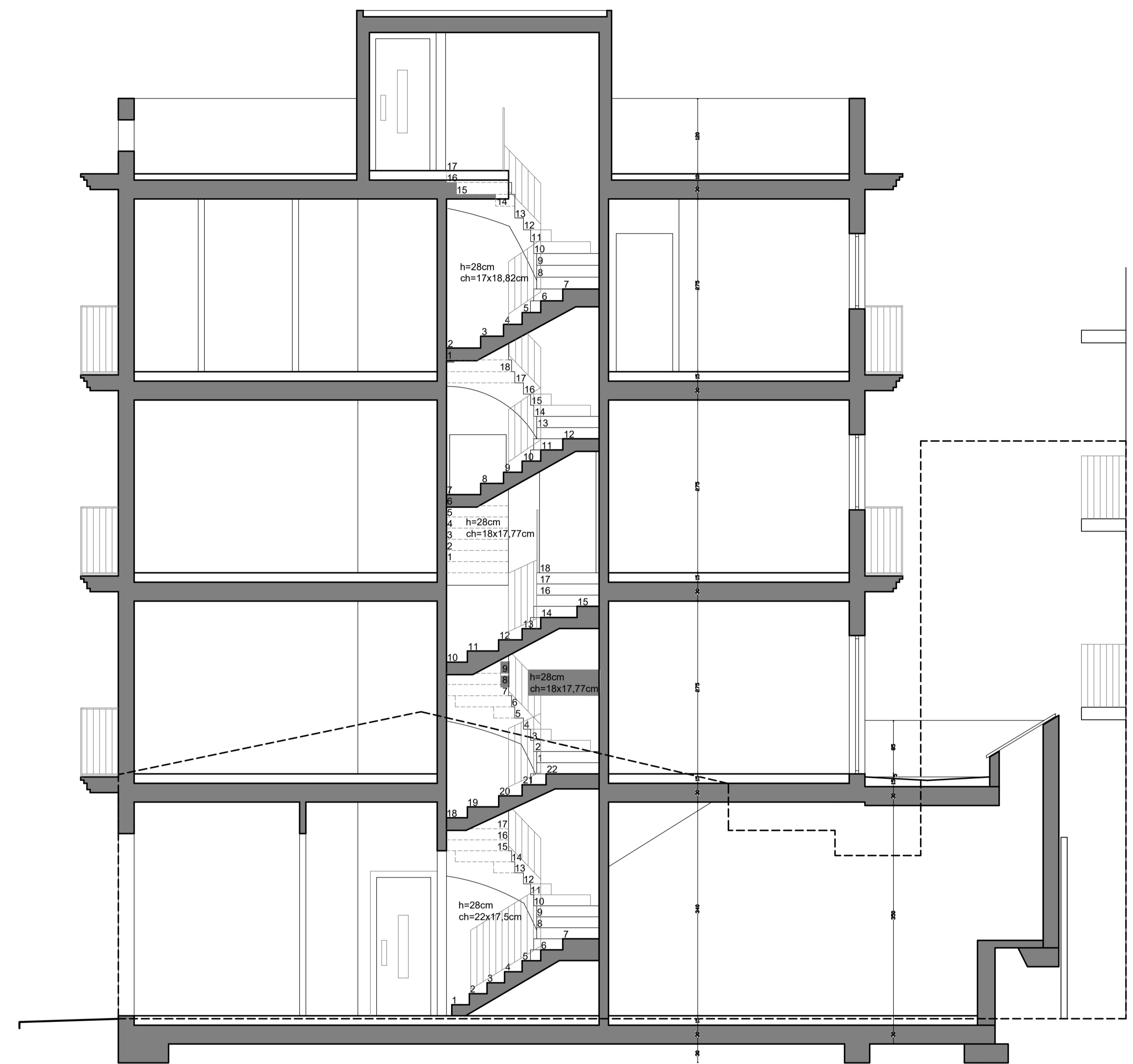
SECCIÓN B-B - E:1/50
