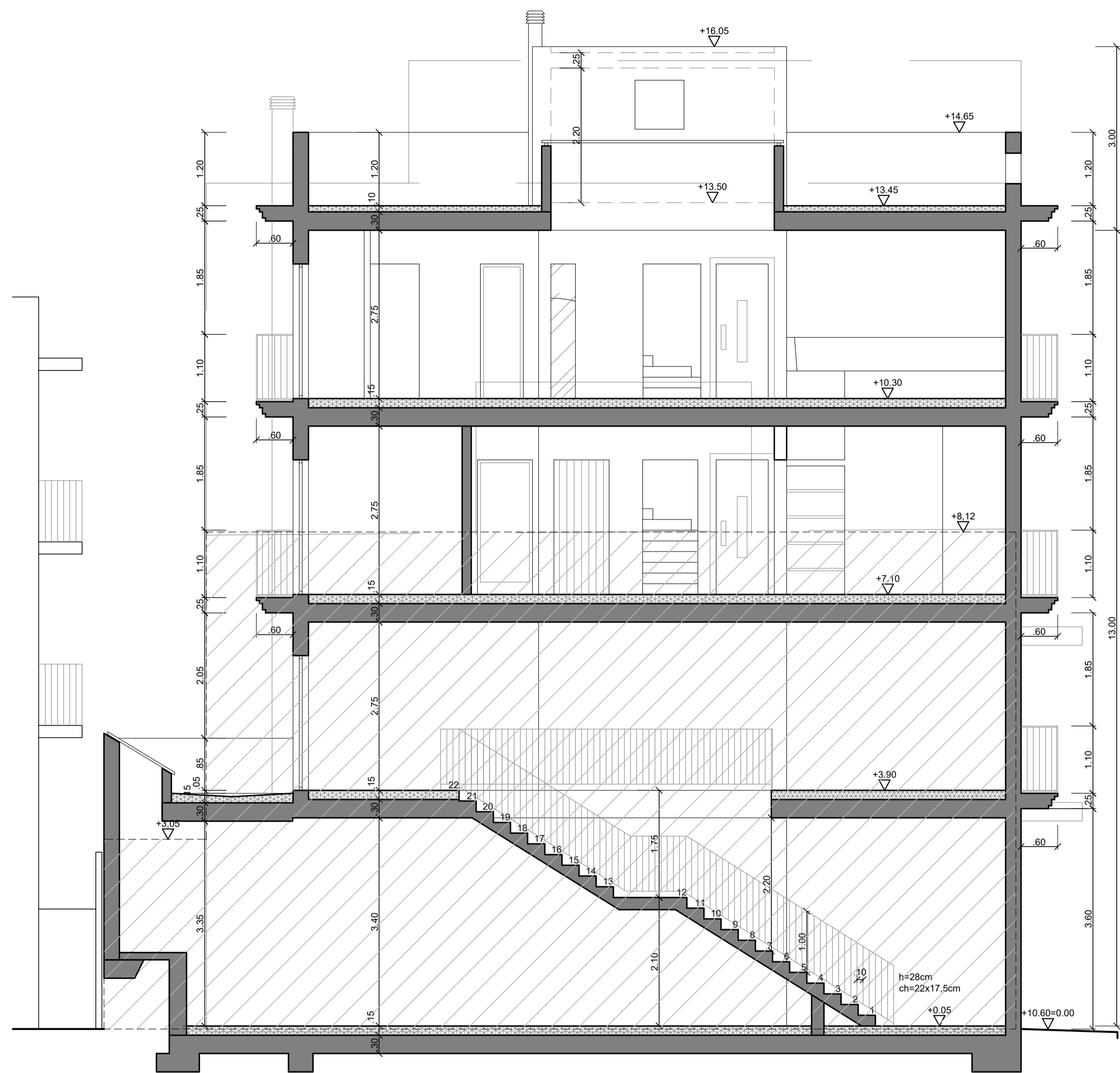
SECCIÓN A-A - E:1/50
