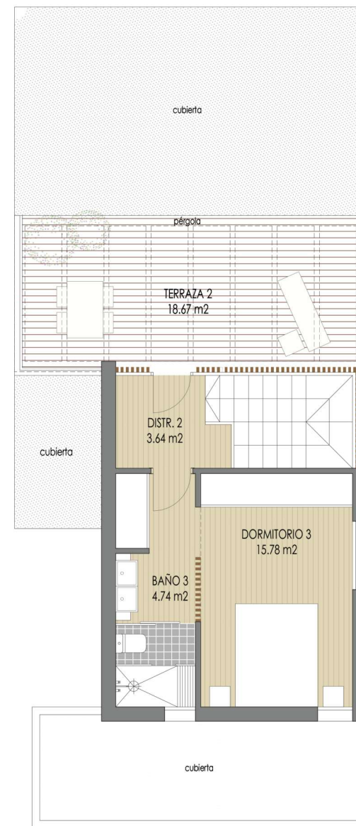
PLANTA PRIMERA
