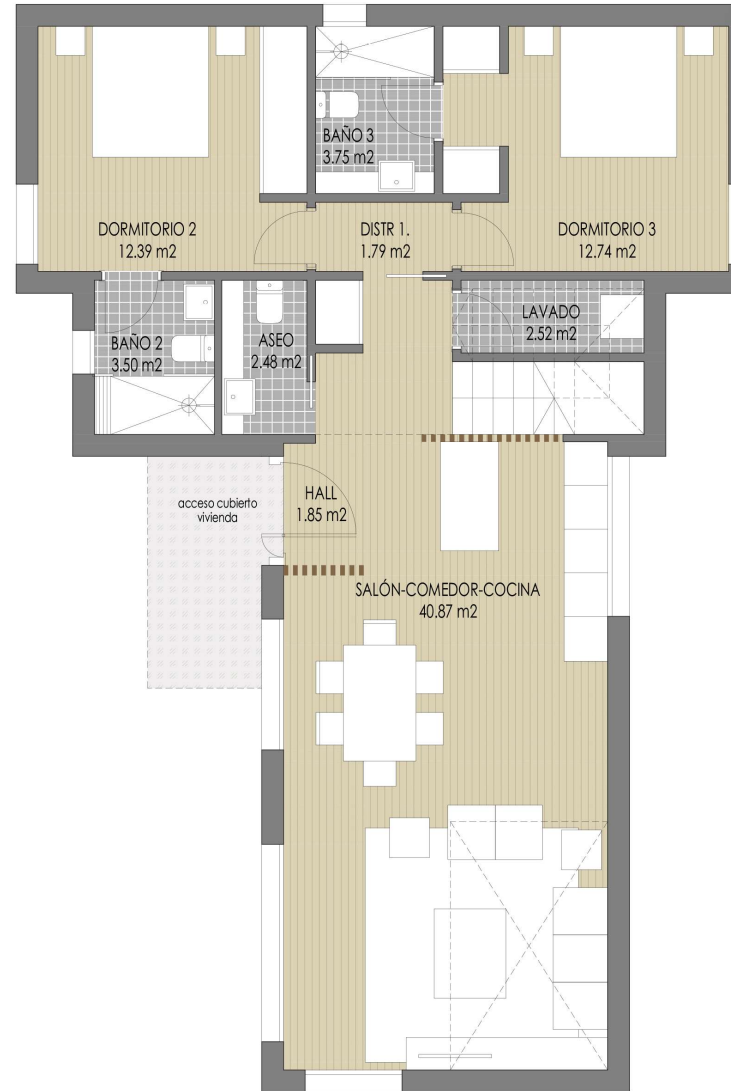
PLANTA BAJA
