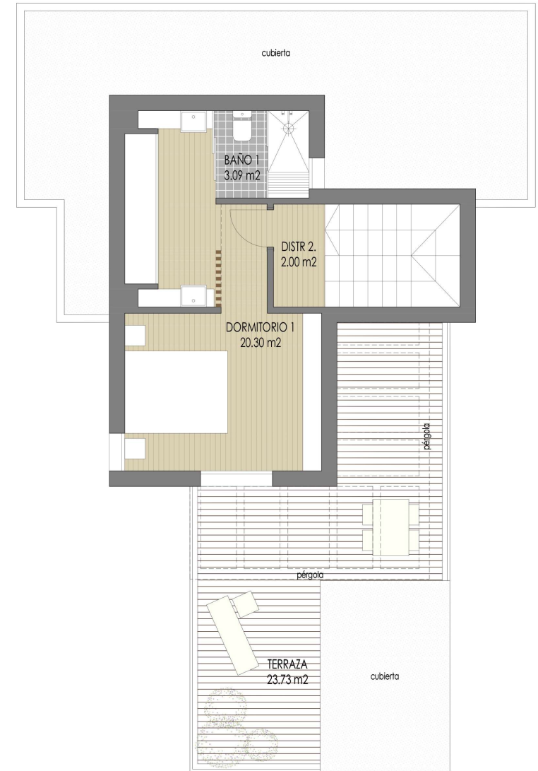
PLANTA PRIMERA
