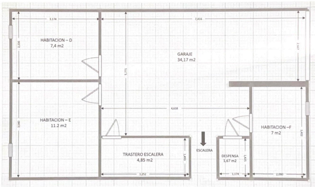
PLANTA SEMISOTANO – 66,29m 2
