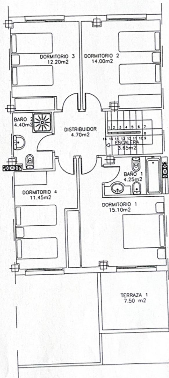
PLANTA PRIMERA
