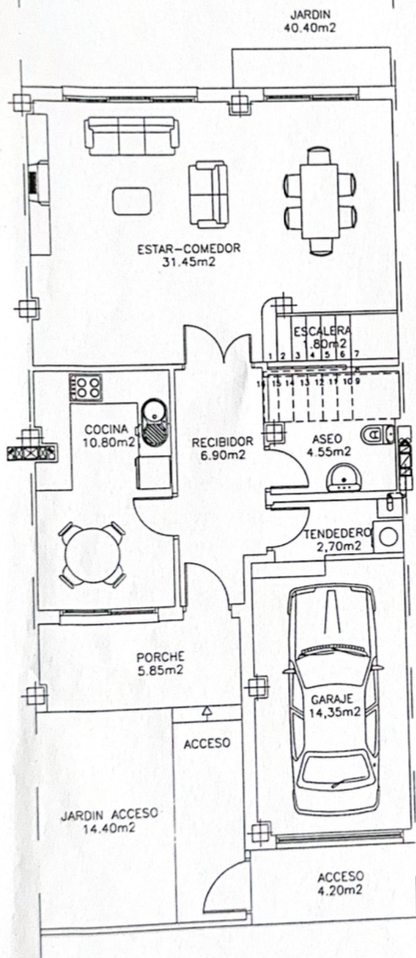
PLANTA BAJA
