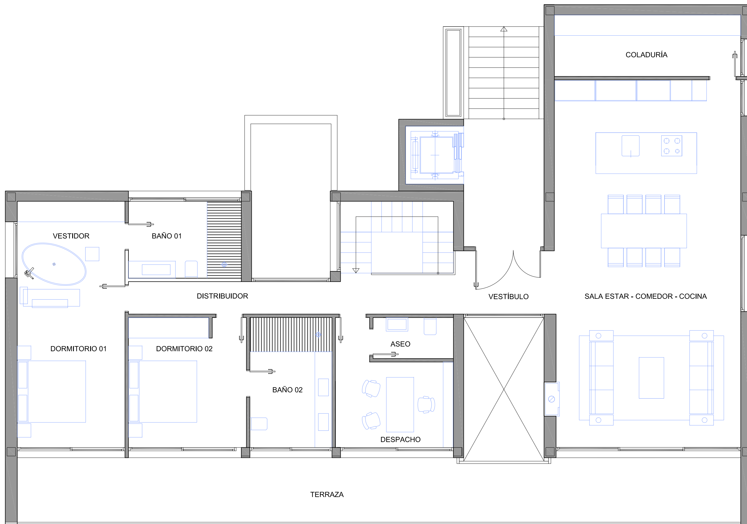
PLANTA PISO
