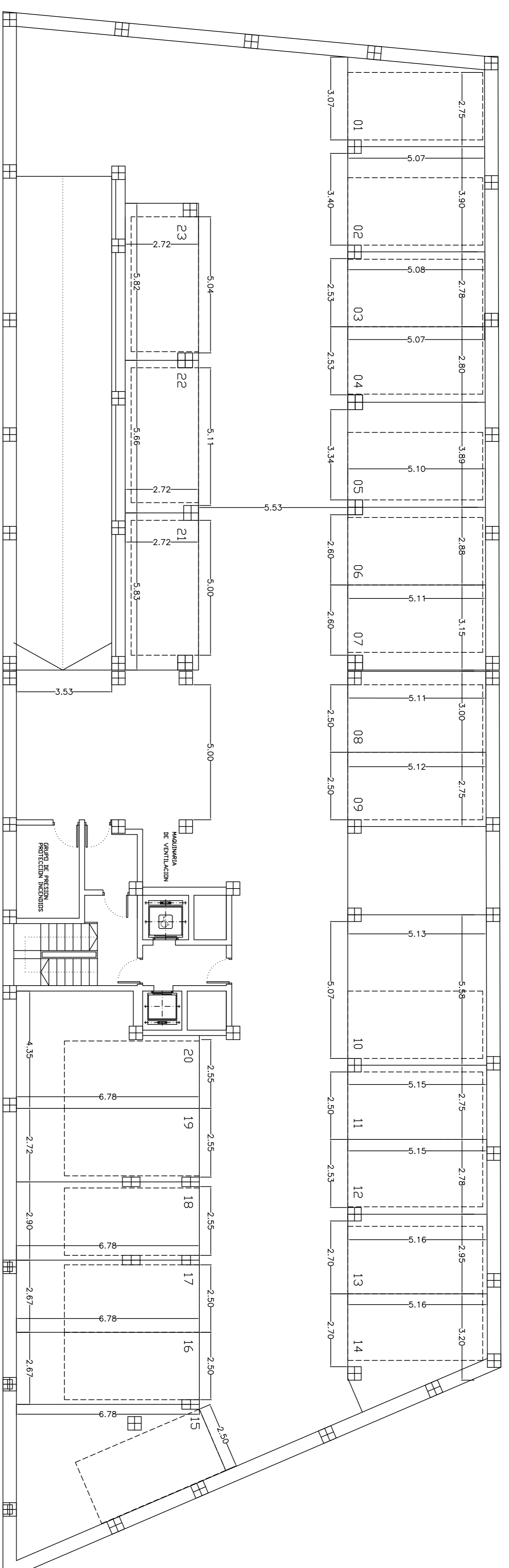
PLANTA SOTANO-GARAJE -1
