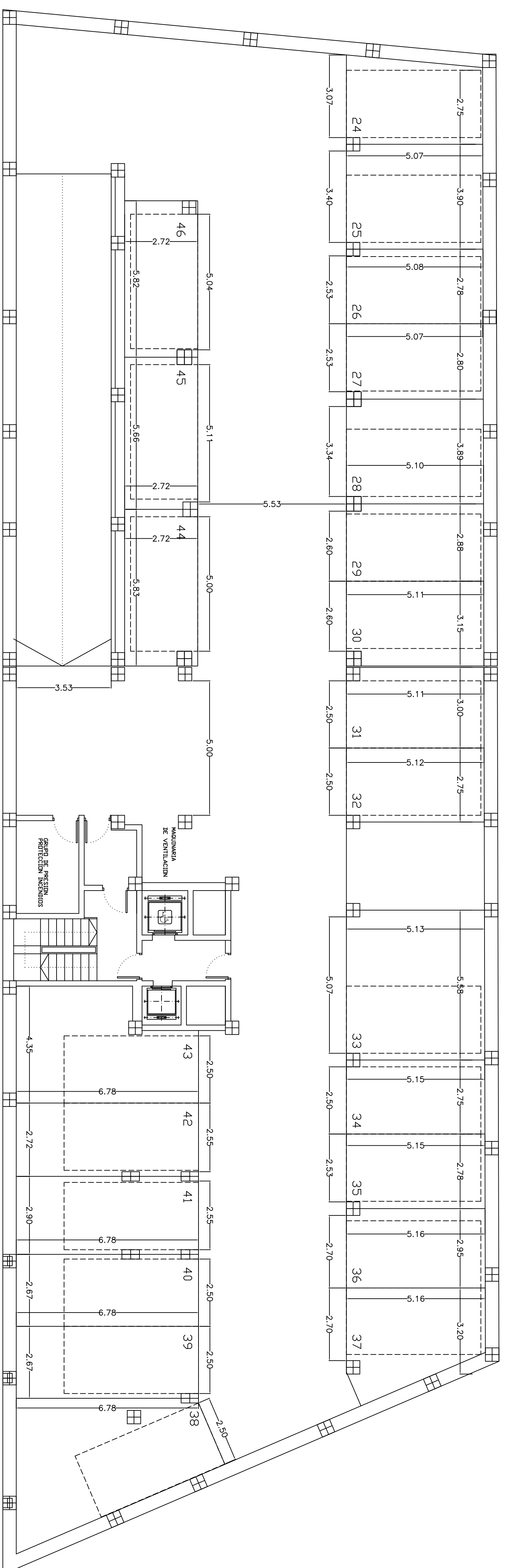
PLANTA SOTANO-GARAJE -2
