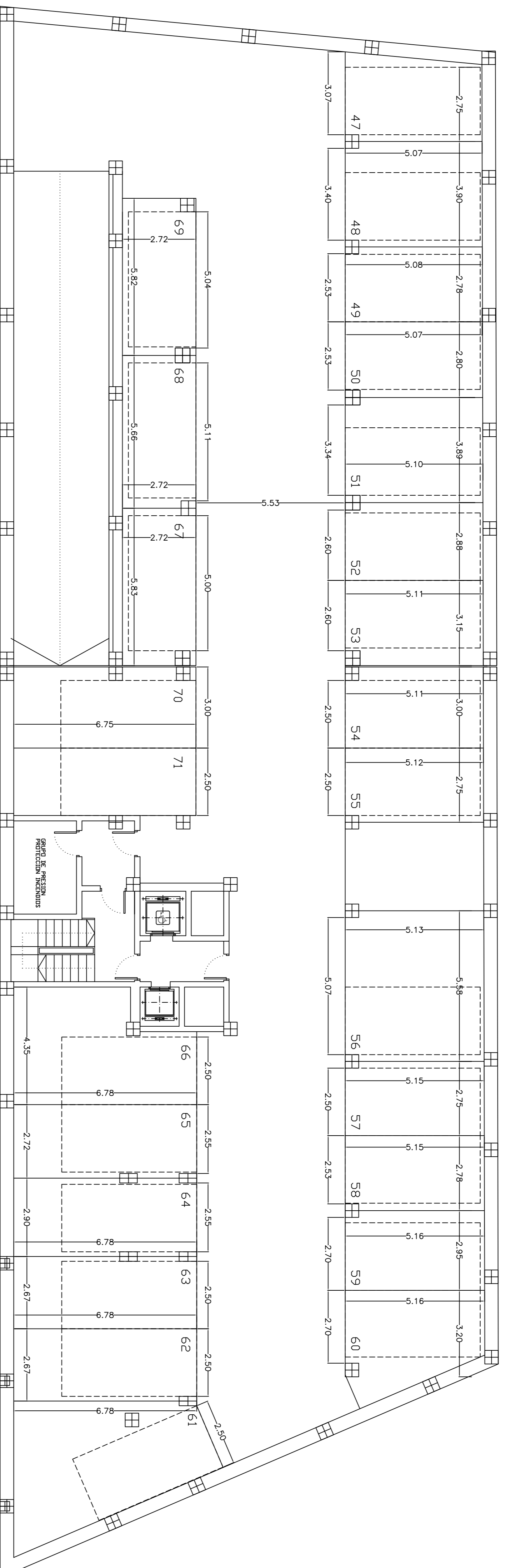
PLANTA SOTANO-GARAJE -3
