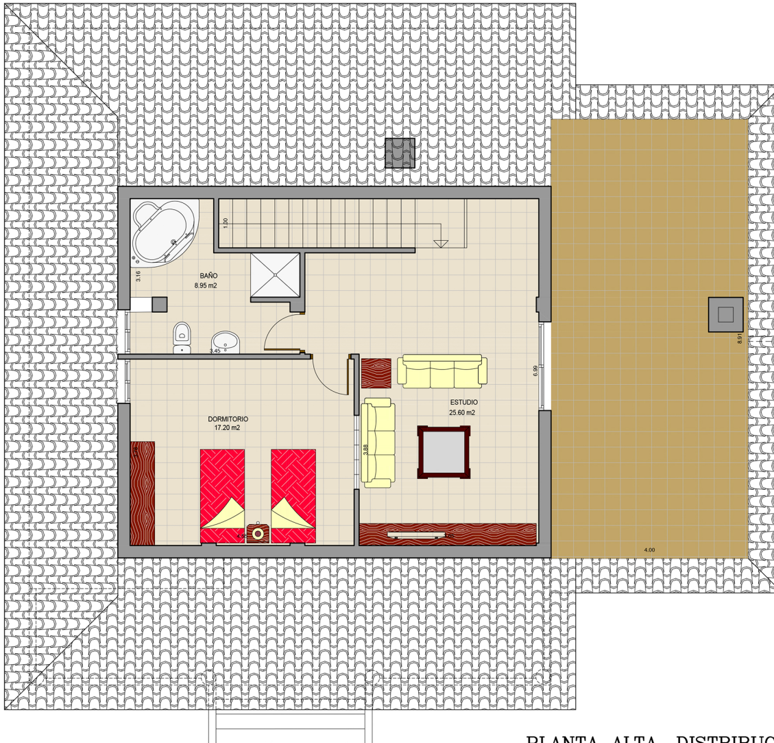
PLANTA ALTA. DISTRIBUCION, COTAS, SUPERFICIES
