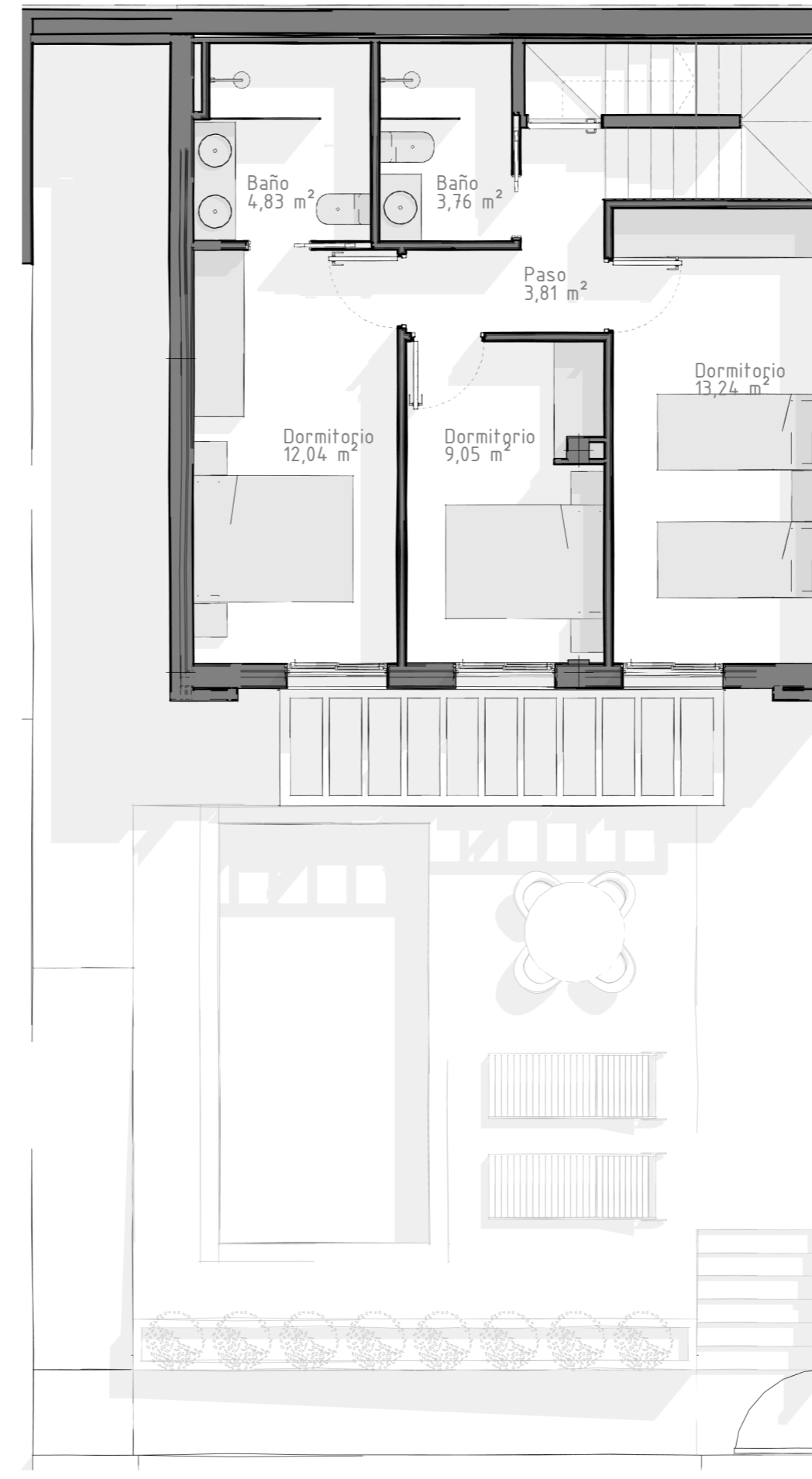
10.Viv. Unifamiliar. Planta 1ª
