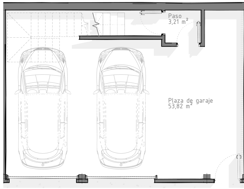
2.Viv. Unifamiliar. Sótano
