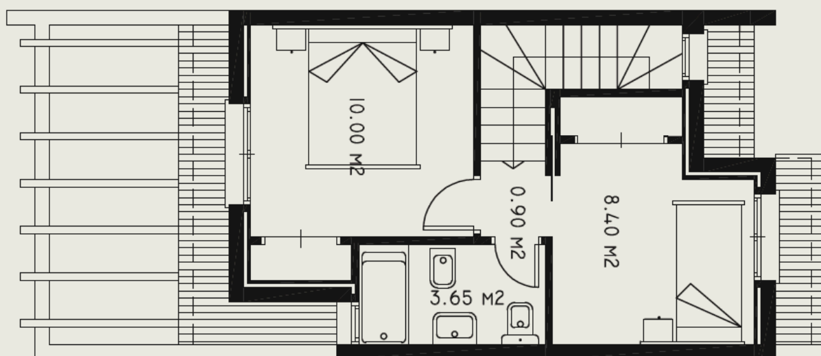
PLANTA ALTA
