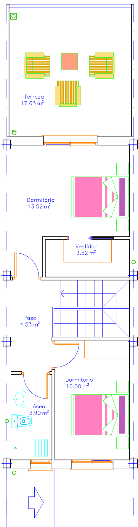
PLANTA 1, S.C.: 47.17M2
