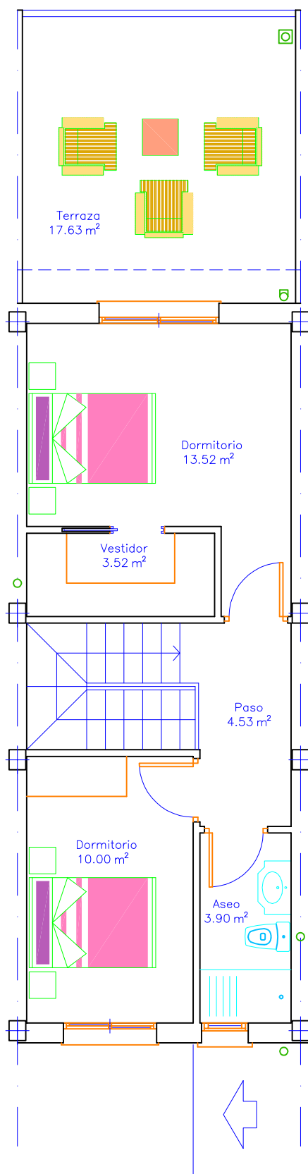
PLANTA 1, S.C.: 47.17M2
