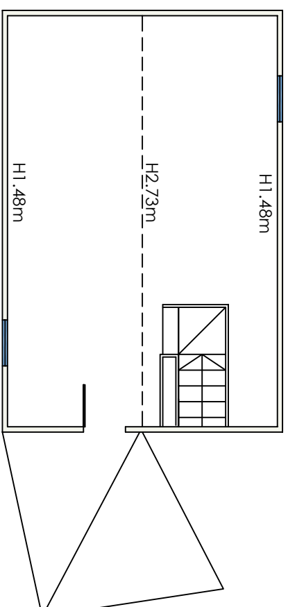
PLANTA BAJO CUBIERTA 54m 2 construidos
