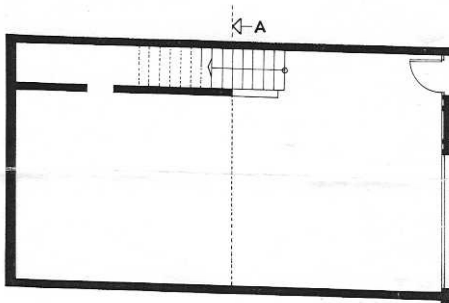
PLANTA SEMISOTANO
