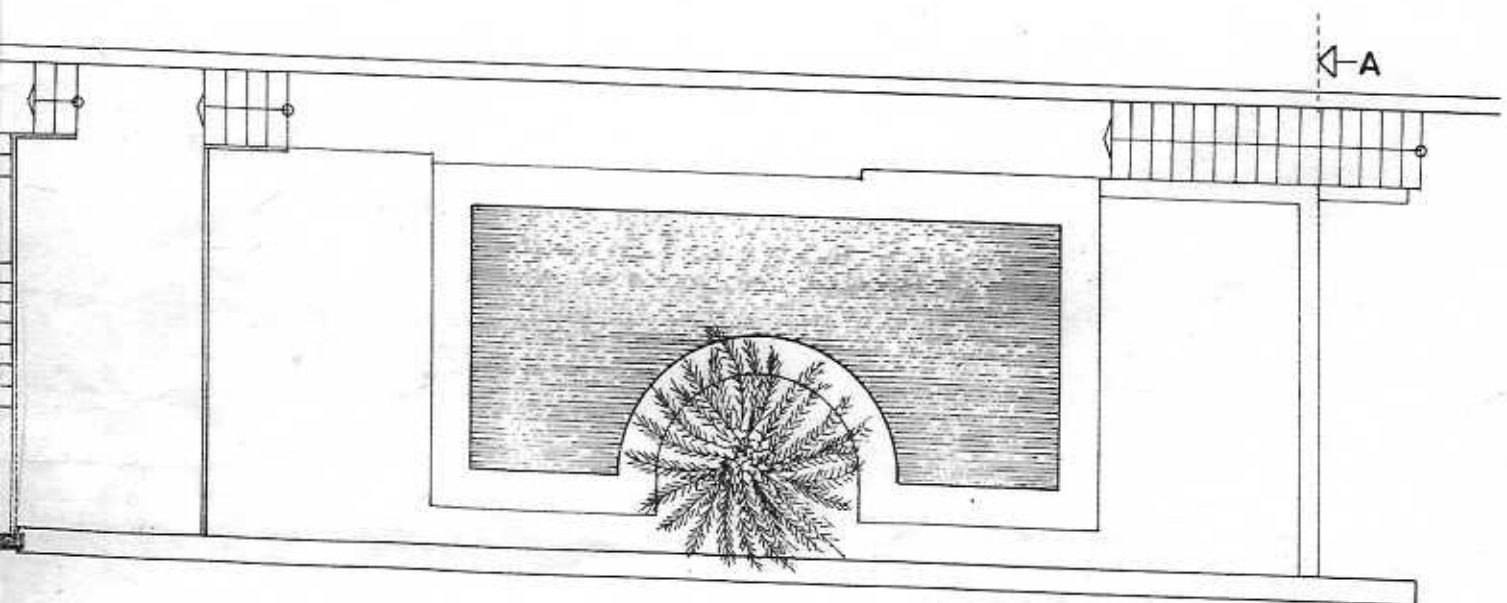
PLANTA SEMISOTANO
