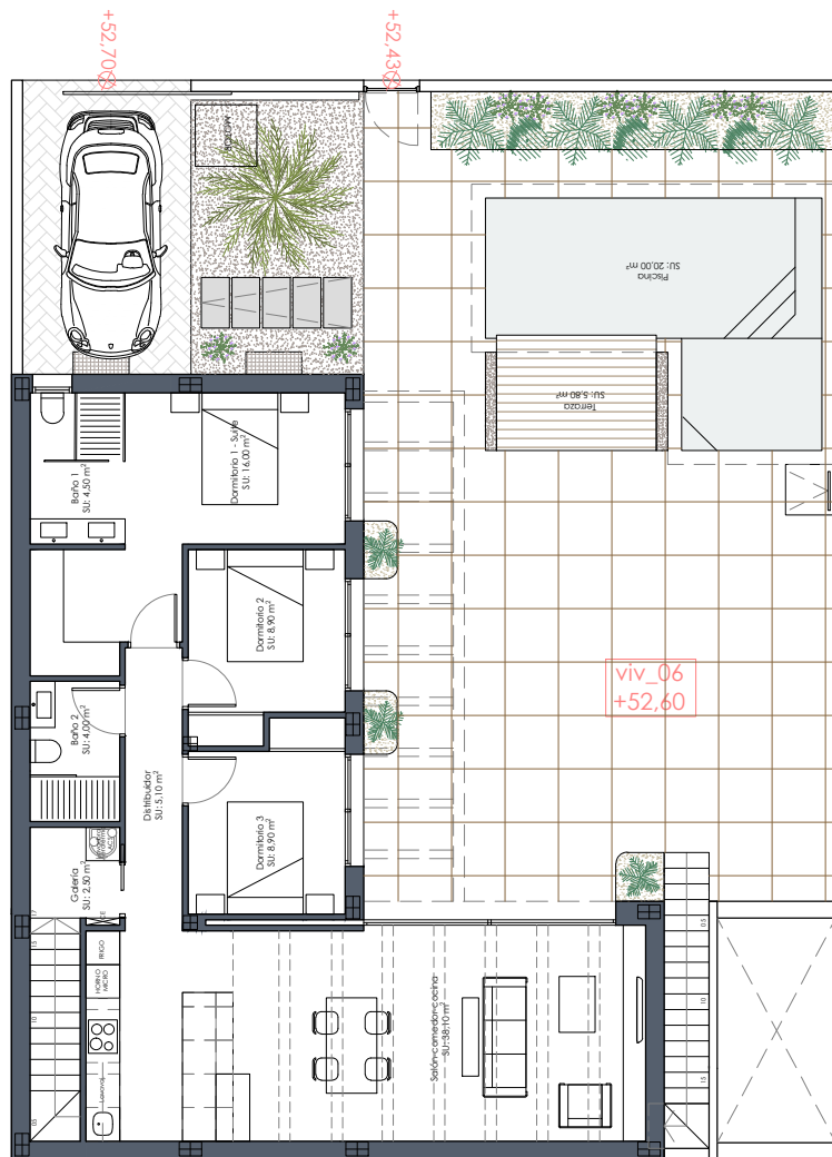
PLANTA BAJA
