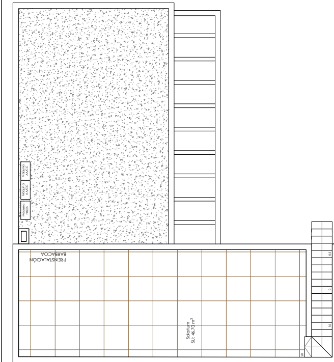
PLANTA CUBIERTA
