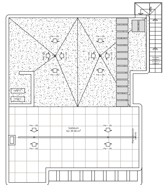
PLANTA SOLARIUM
