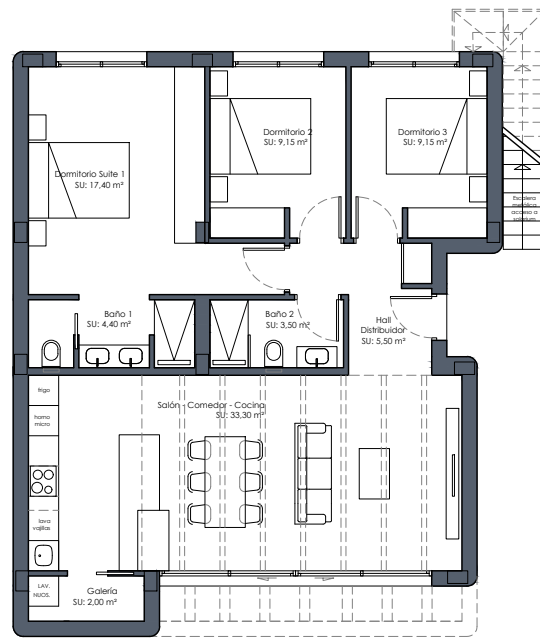
PLANTA BAJA
