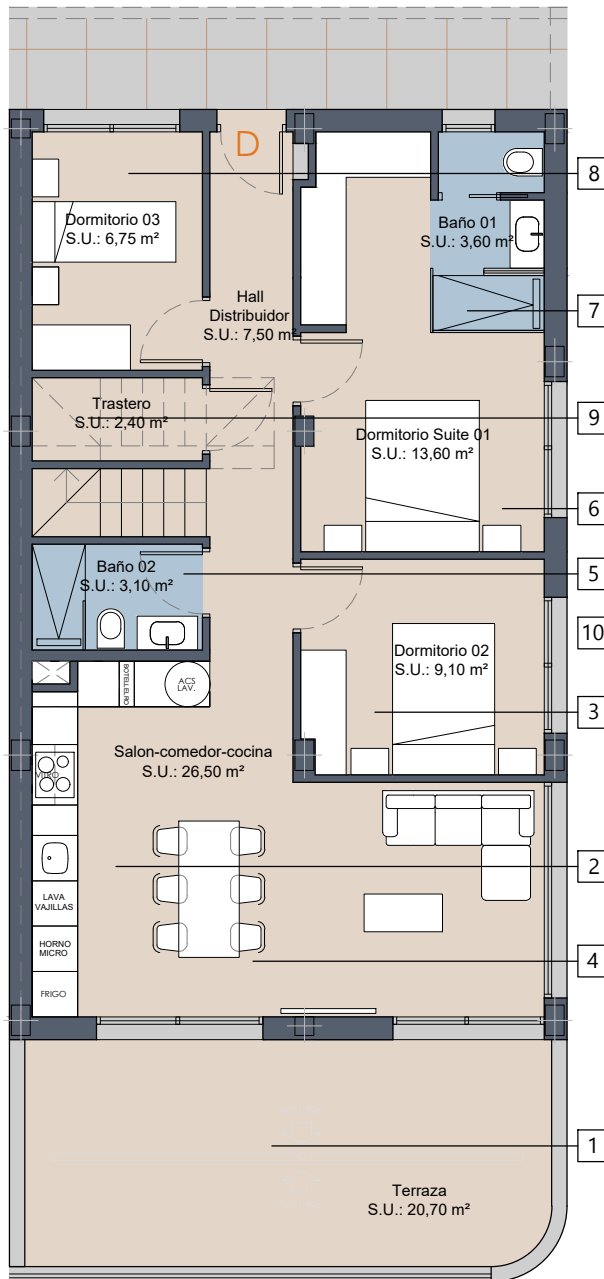
PLANTA SEGUNDA
