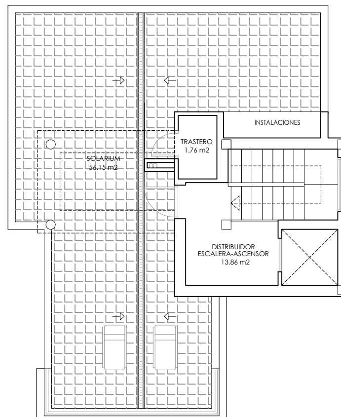
PLANTA CUBIERTA
