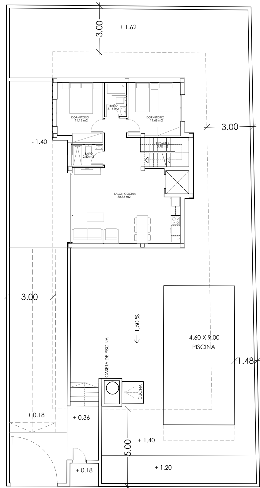
PROPUESTA SOTANO
