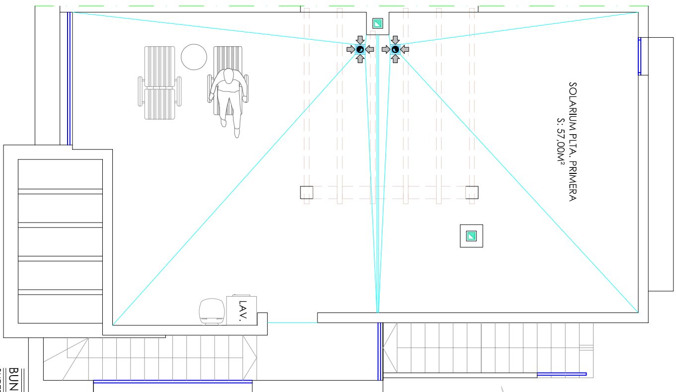
PLANTA DE SOLARIUM
