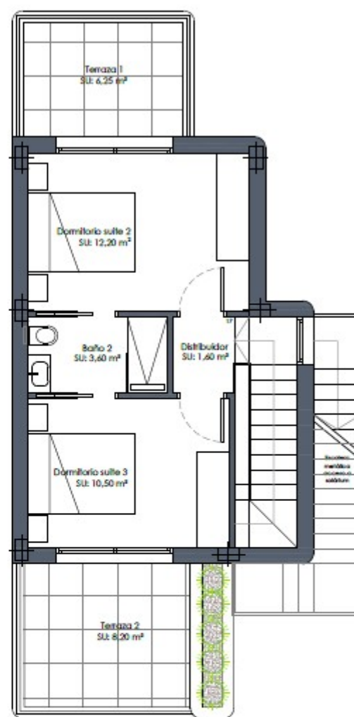
PLANTA PRIMERA
