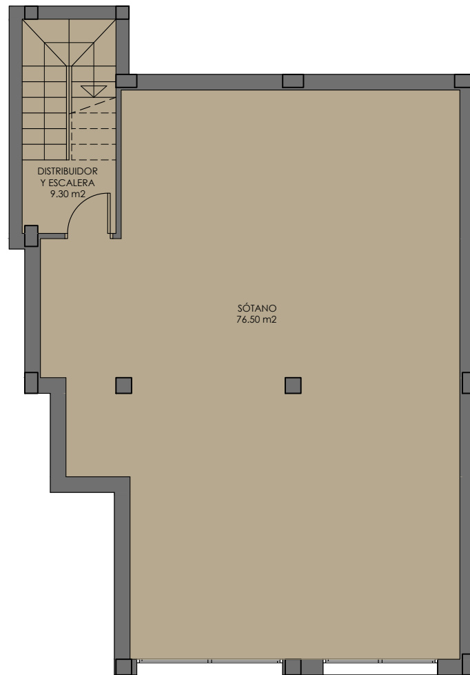
PLANTA SEMISÓTANO
