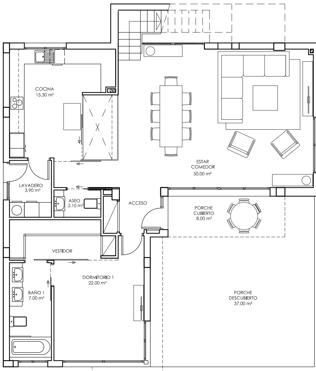
PLANTA BAJA
