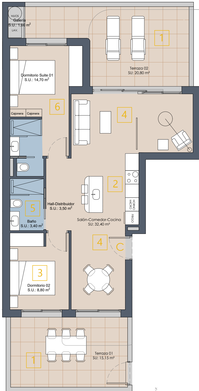
PLANTA BAJA
