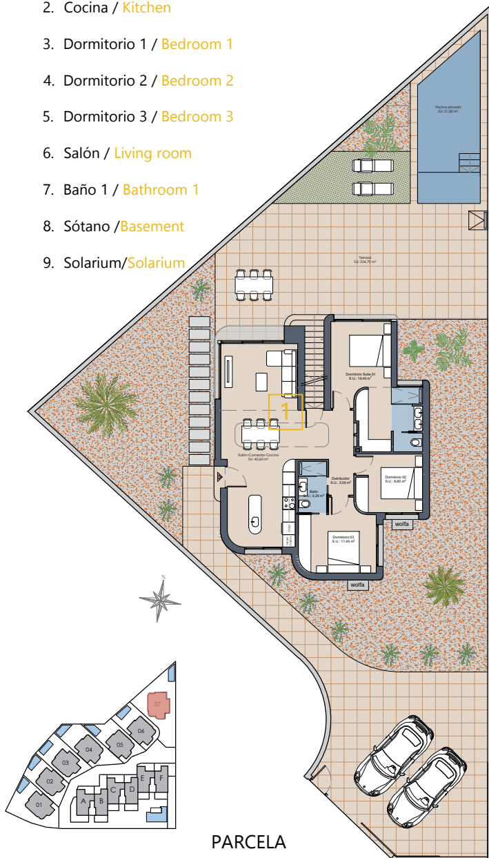
PLANTA BAJA
