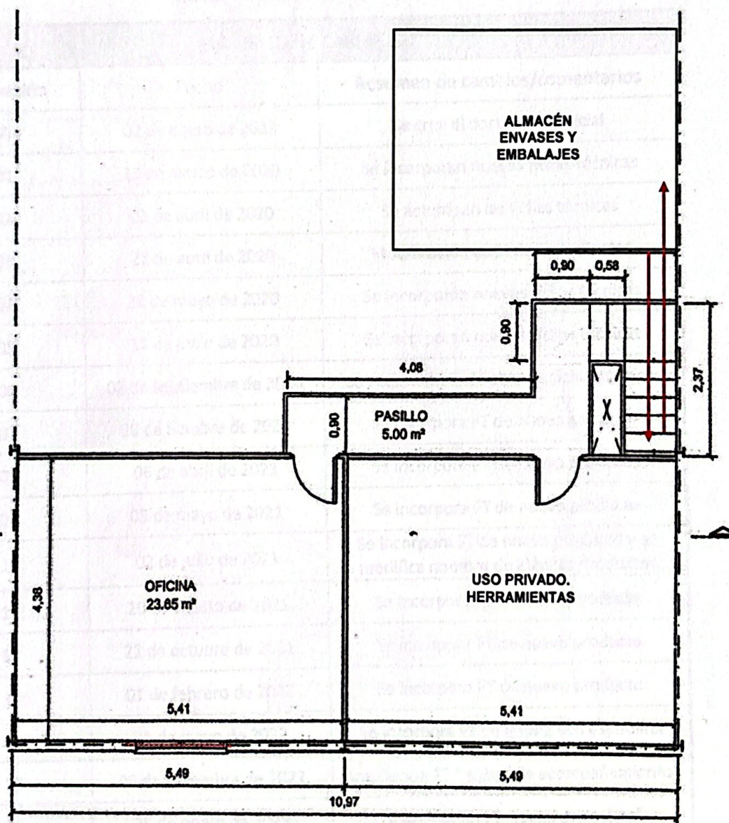
PLANTA ALTA
