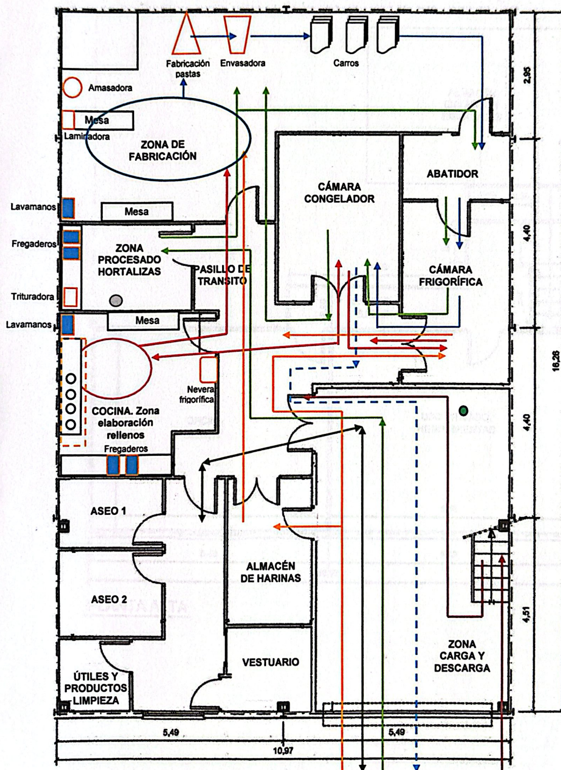
PLANTA BAJA
