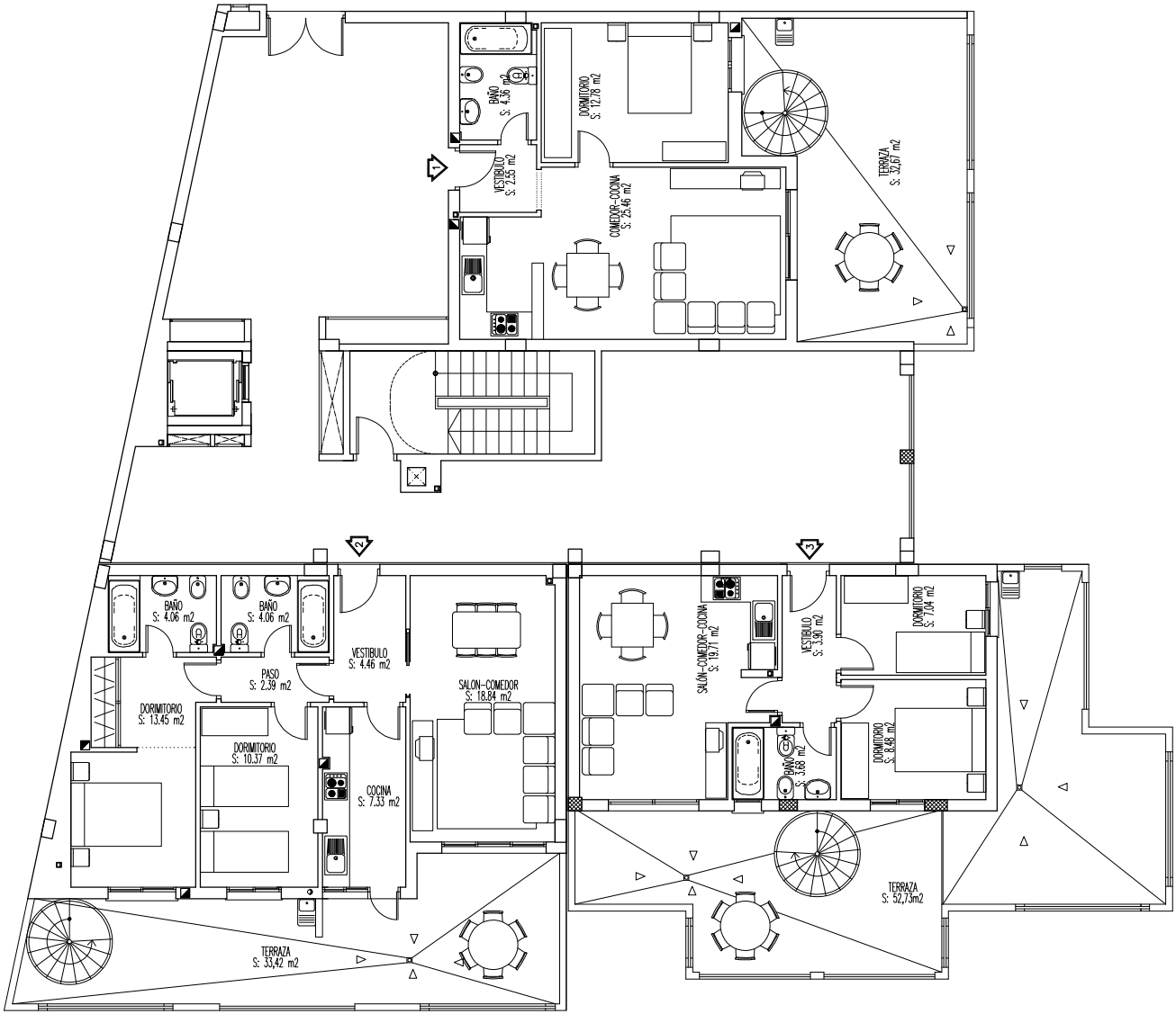
BLOQUE 5 PLANTA TERCERA DISTRIBUCIÓN Y SUPERFICIES
