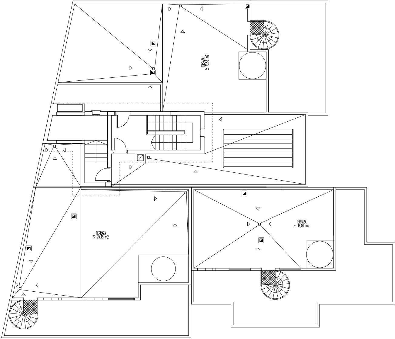
BLOQUE 5 PLANTA CUBIERTA DAN: CUBIERTA NO TRANSITABLE DAT: CUBIERTA TRANSITABLE NOTA: TODAS LAS PENDIENTES DE LA CUBIERTA SERÁN COMO MÍNIMO DEL 2%
