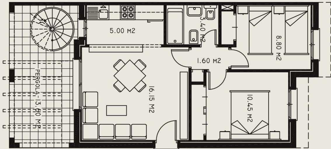
PLANTA BAJA
