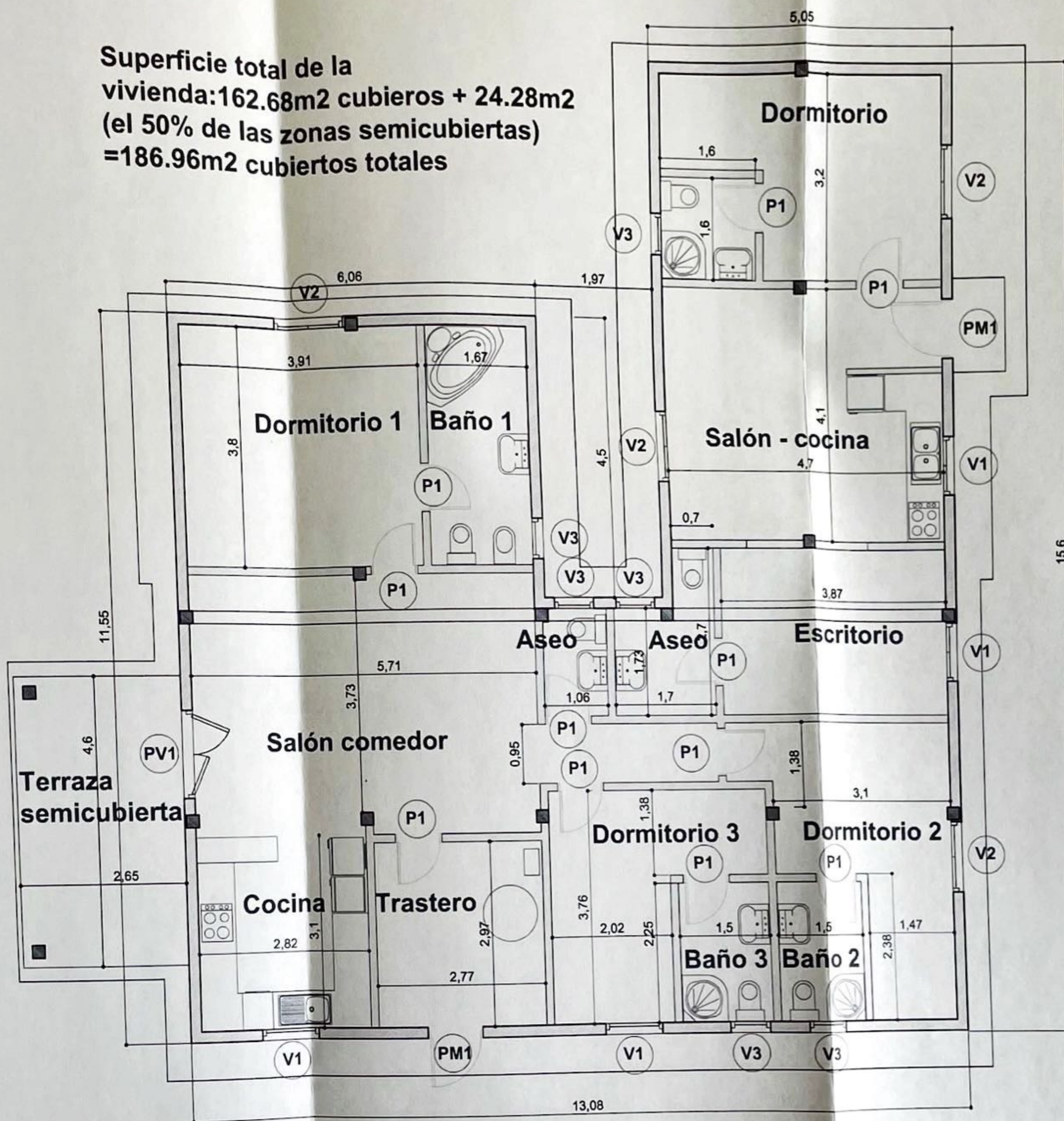
PLANTA DE DISTRIBUCIÓN
