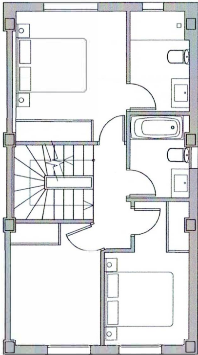
PLANTA PRIMERA
