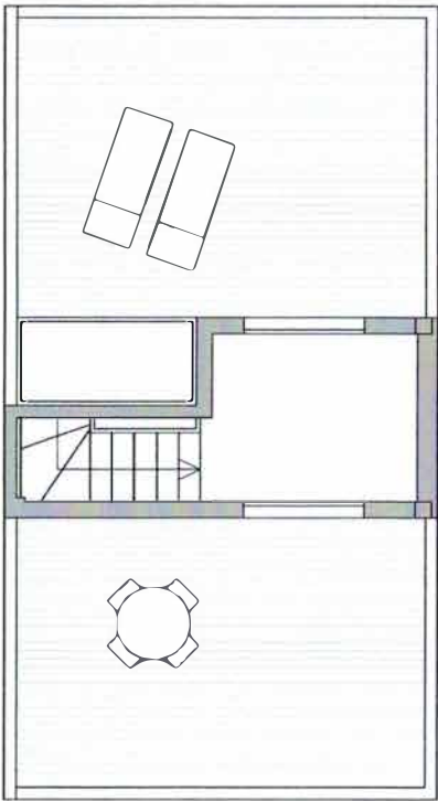
PLANTA CUBIERTA
