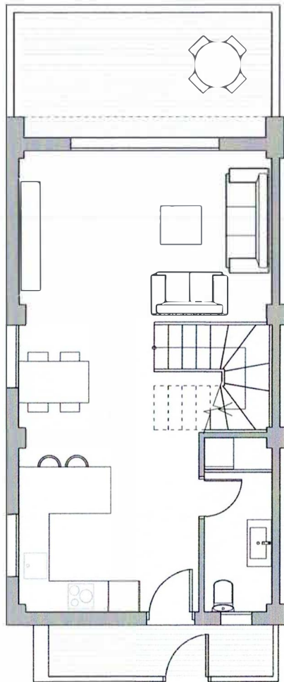
PLANTA BAJA
