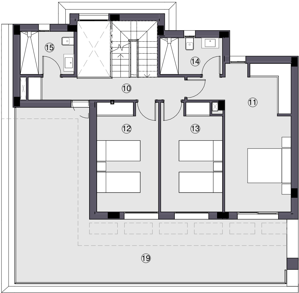
PLANTA PRIMERA / FIRST FLOOR
