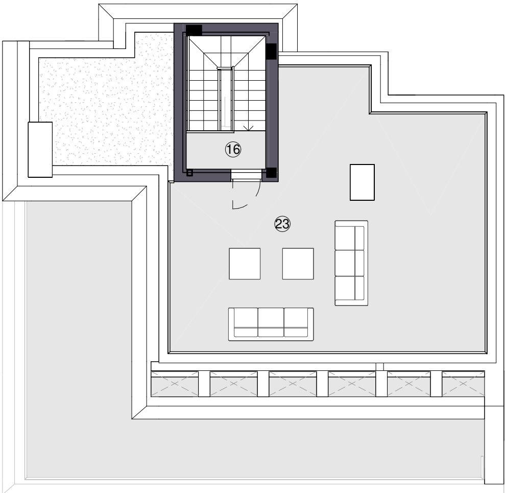
PLANTA SEGUNDA / SECOND FLOOR
