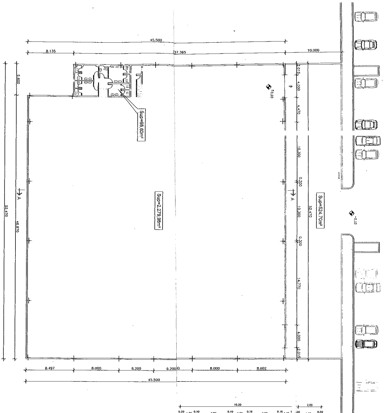
PLANTA BAJA. COTAS
