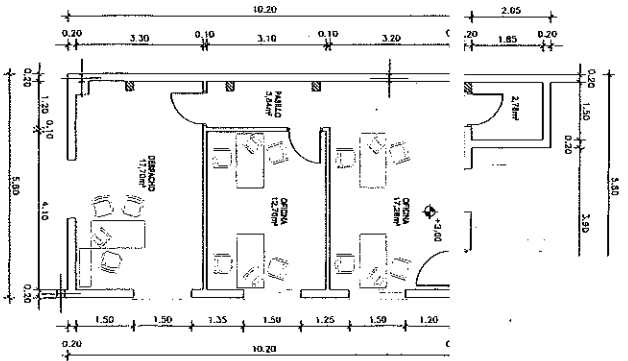
PLANTA ALTA. COTAS
