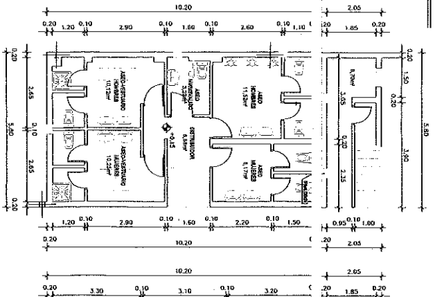
PLANTA BAJA. COTAS
