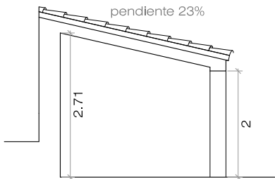
Secció transversal
