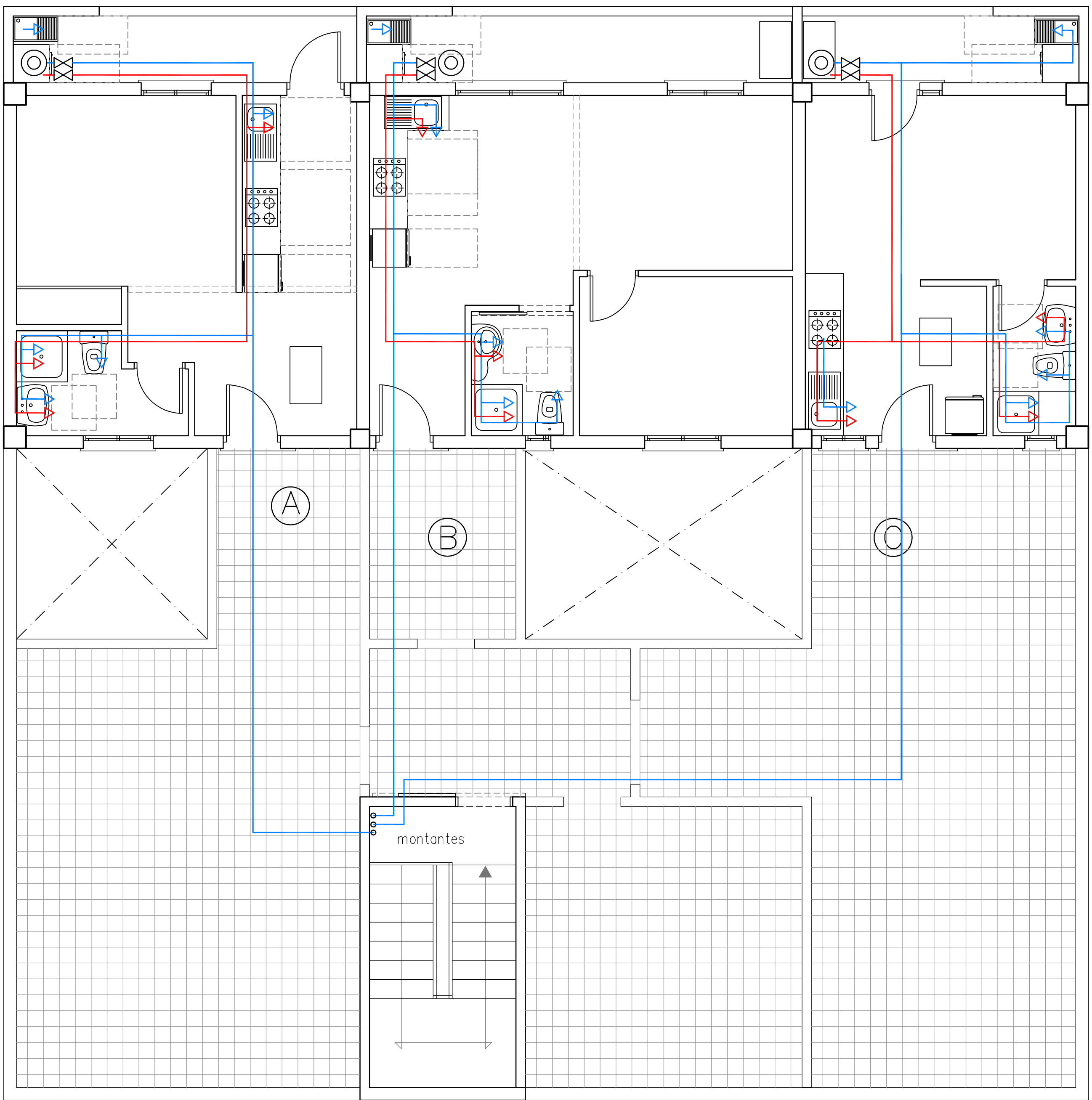
PLANTA CUBIERTA esquema fontaneria
