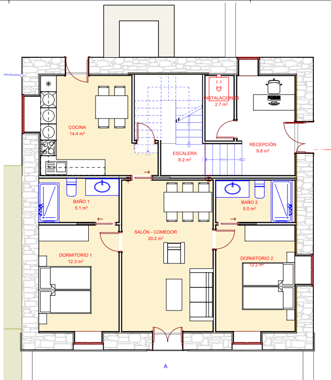
Planta Baja - 1:50
