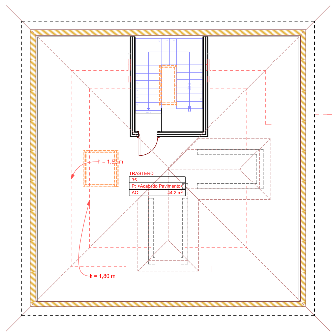
Bajocubierta - 1:50
