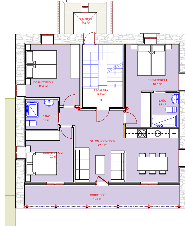
Planta 2 - 1:50
