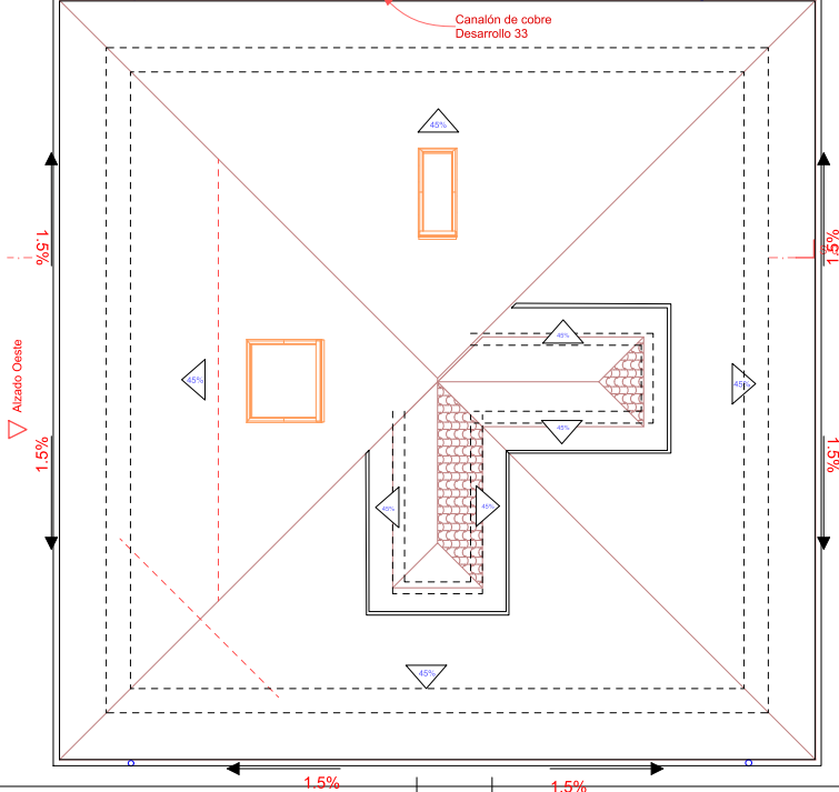
Planta 1 - 1:50
