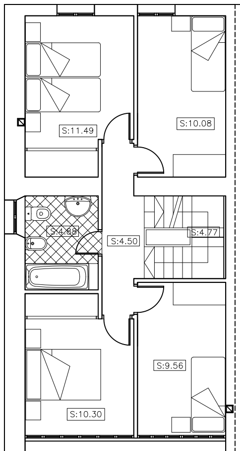
PLANTA PRIMERA
