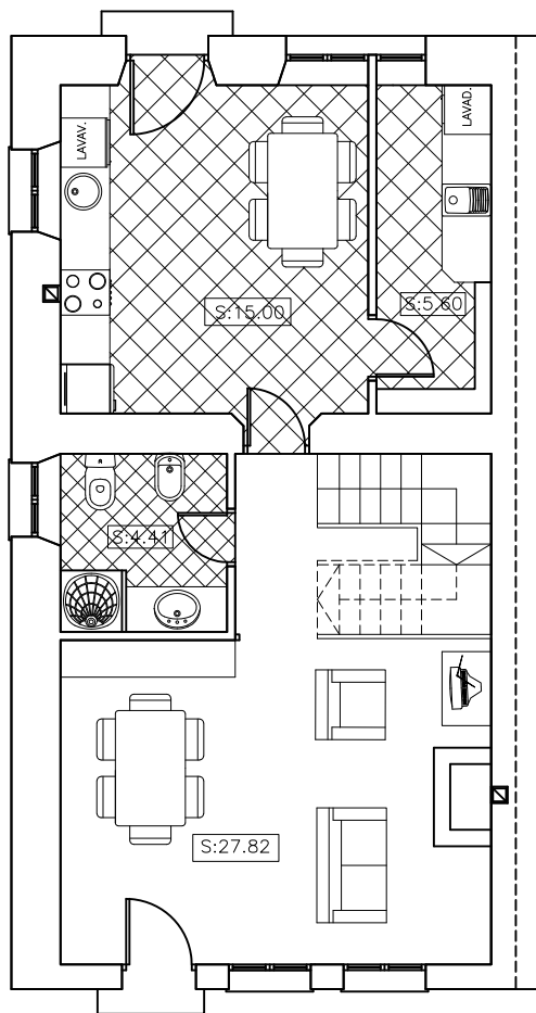
PLANTA BAJA
