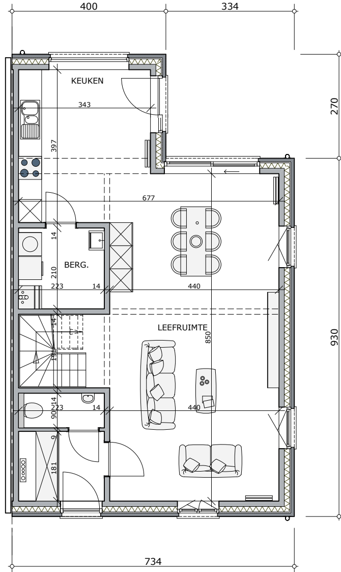
GELIJKVLOERS Opp.= 79.06 m 2
